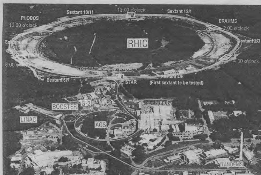
अमेरिकाको क्यालिफोर्नियाको ब्रूकहेभनस्थित हिक (RHIC) नामक कण परीक्षणशाला
