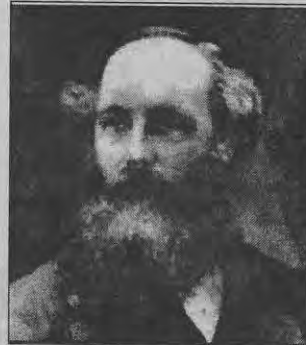
जेम्स म्याक्सवेल
